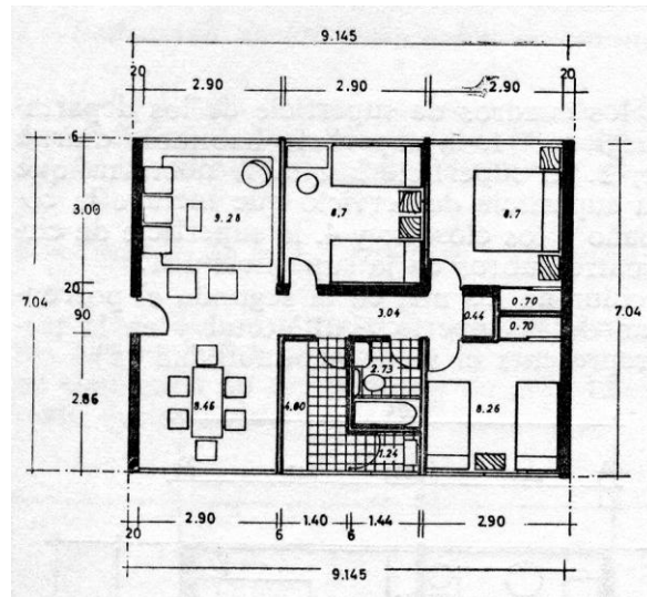
Figura 5.-Departamento tipo B: 3 dormitorios, 6 camas. "Villa Italia".
