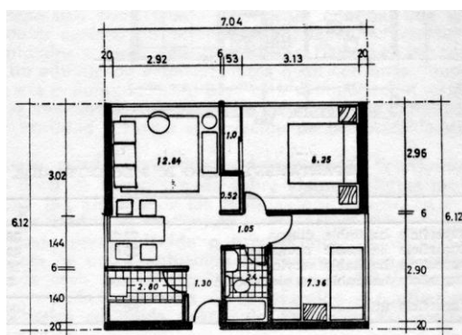
Figura 4.-Departamento Tipo A: 2 dormitorios, 4 camas. "Villa Italia".
